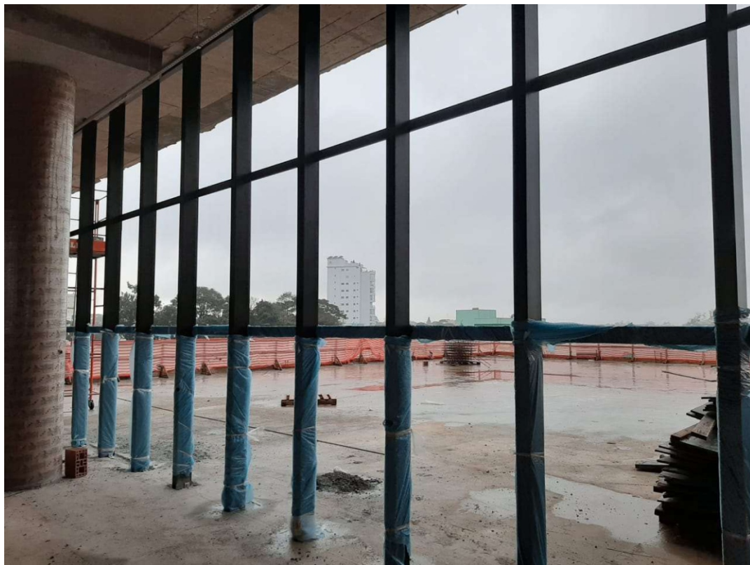
Montagem PV 10 e PV 16 – 2º Pav
