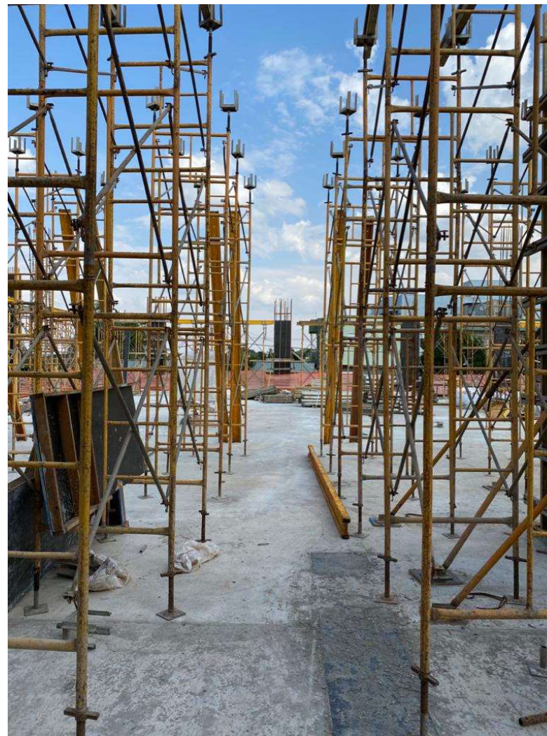
Montagem do Cimbramento da Laje 2º Pav
