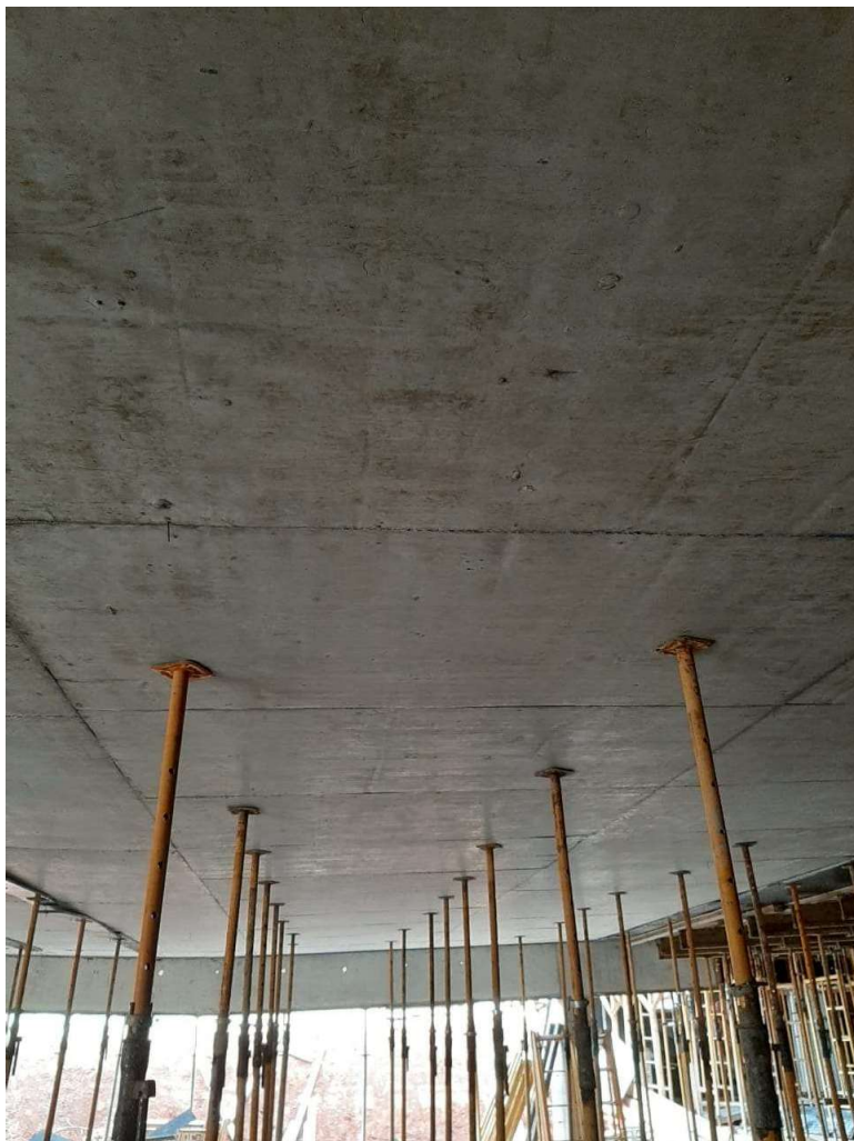
Laje do Térreo Desformada
